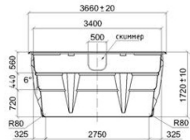
Вид - А
